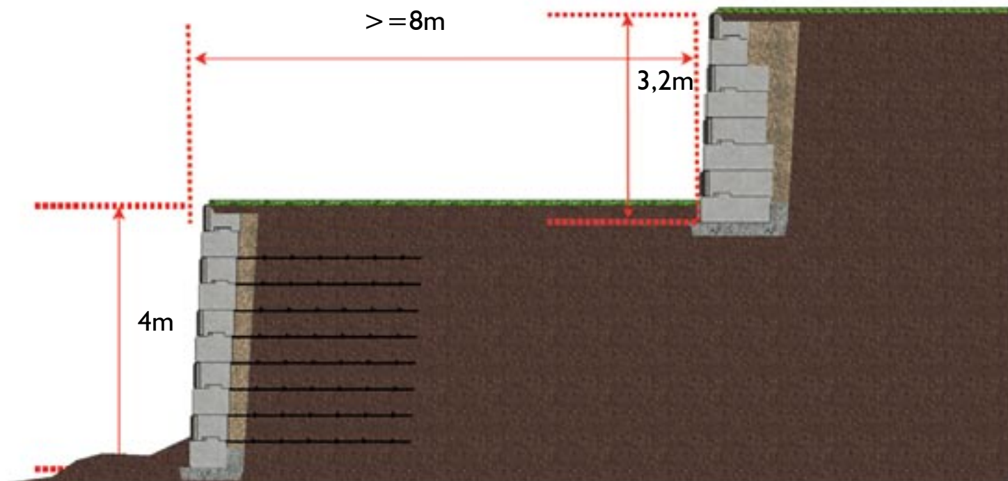
Eksempel på terrassemur
